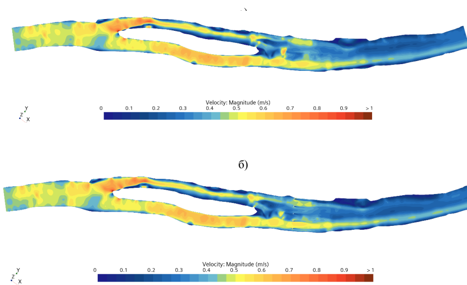
Рис. 4. Скалярное распределение поверхностных скоростей а) естественное состояние; б) проектное состояние.
