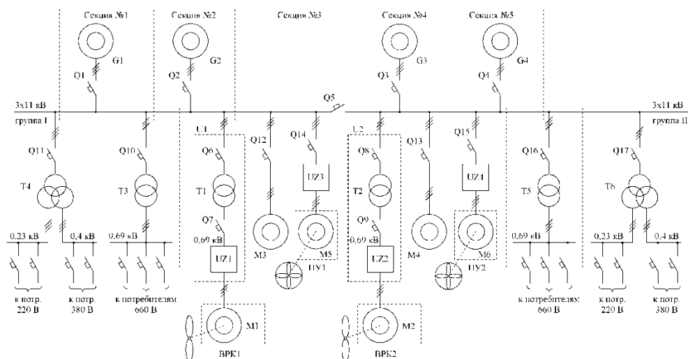
Рис. 2. Однолинейная схема единой судовой электроэнергетической системы
