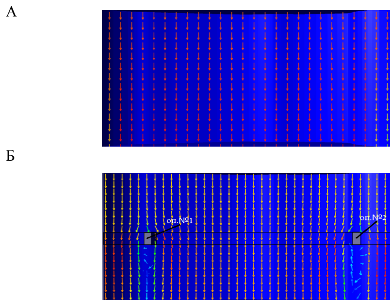
Рис. 5. Поведение потока в створе мостового перехода в II зоне.
