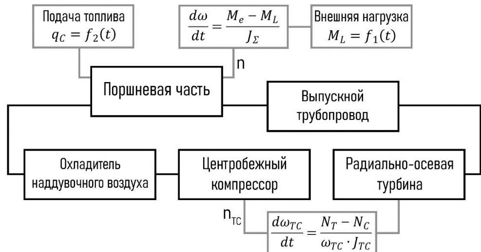
Рис. 1. Структурная схема термогазодинамической системы
