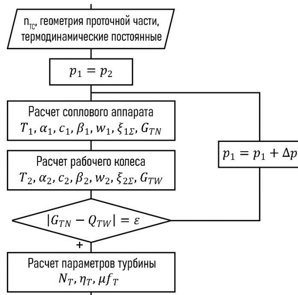
Рис. 4. Блок-схема расчета радиально-осевой турбины: p_1 – давление между сопловым аппаратом и рабочим колесом; p_2 – давление на выходе из турбины; G_{TN} и G_{TW} – массовые расходы газа через сопловой аппарат и рабочее колесо
