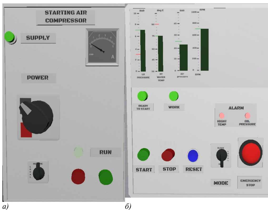
Рис. 6. Местный пульт управления: а) компрессором, б) двигателем
