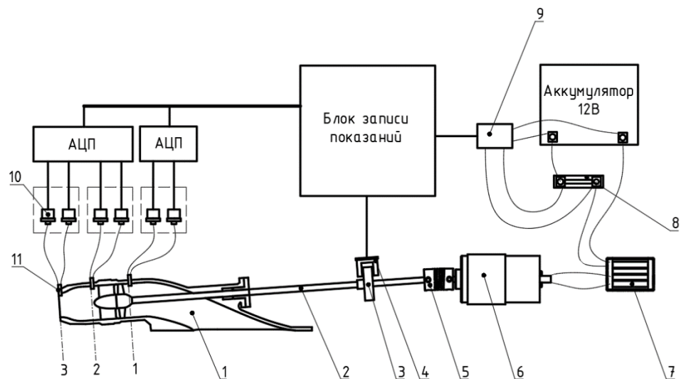
Рис. 4. Схема измерительного комплекса: 1 – водометный движитель; 2 – валопровод; 3 – щелевой диск; 4 – оптический датчик частоты вращения; 5 – соединительная муфта; 6 – электродвигатель; 7 – регулятор мощности двигателя; 8 – токоизмерительный шунт; 9 – вольтамперметр; 10 – датчики давления; 11 – измерительные трубки
