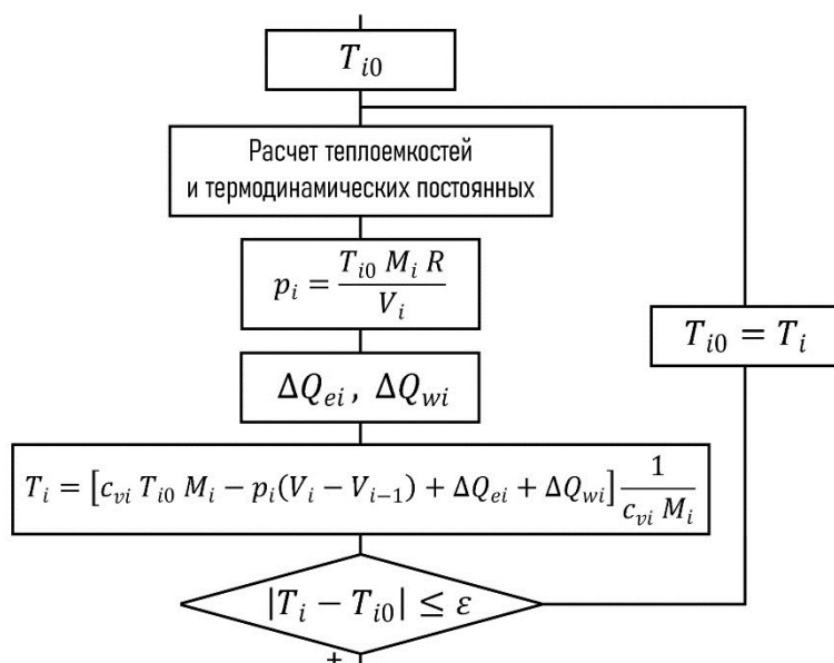
Рис. 2. Блок-схема расчета процесса в цилиндре:
