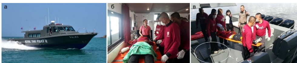
Рис. 10. Катер пр. SB60SAR; а – общий вид; б – отсек paramедицинской помощи; в – кормовая палуба; г – комингс люка на выходе из отсека.
