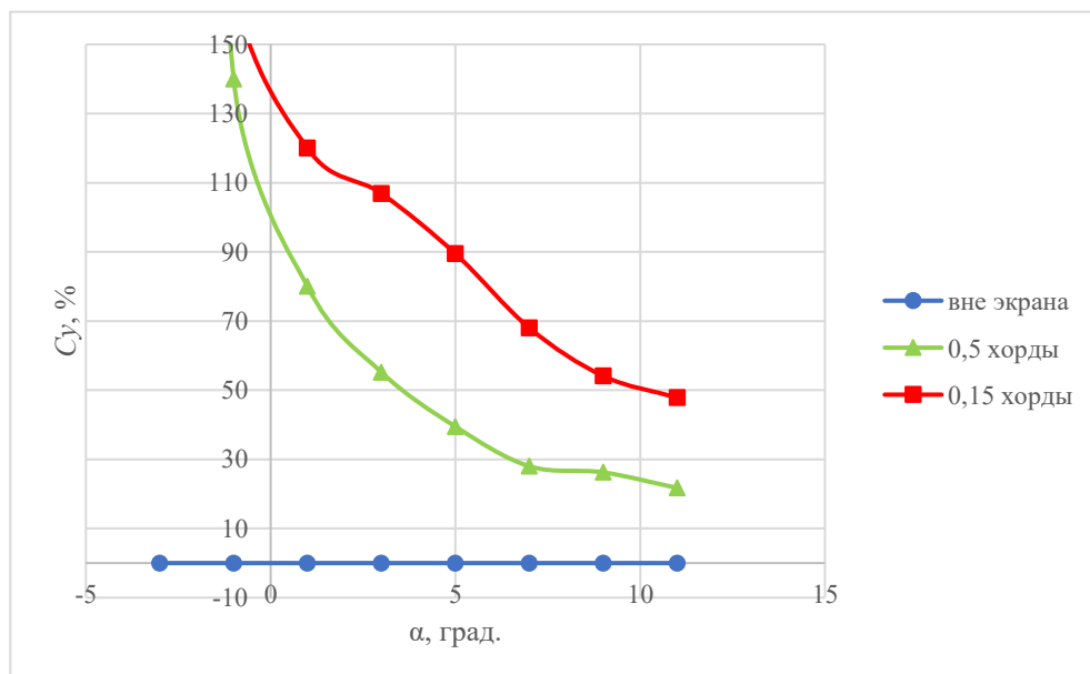
Рис. 15. Кривые зависимости коэффициента подъемной силы от относительной высоты полёта и угла атаки по отношению к значениям крыла вне экрана, ограниченные областью до 150%
