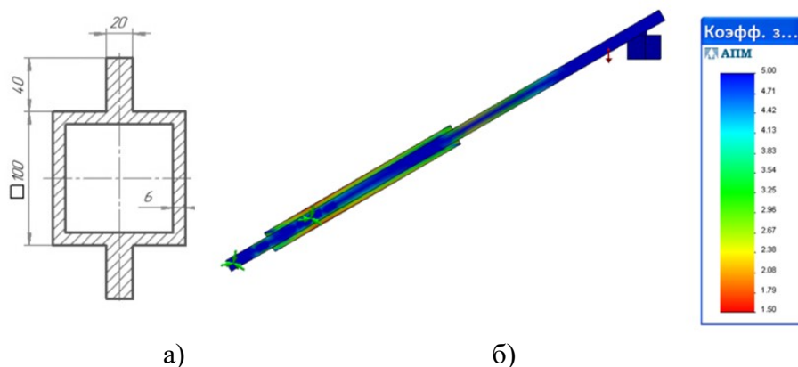
Рис. 5. Сечение профиля рамы с ребрами жесткости: а) и распределение запаса прочности для итоговой конструкции рамы: б)
