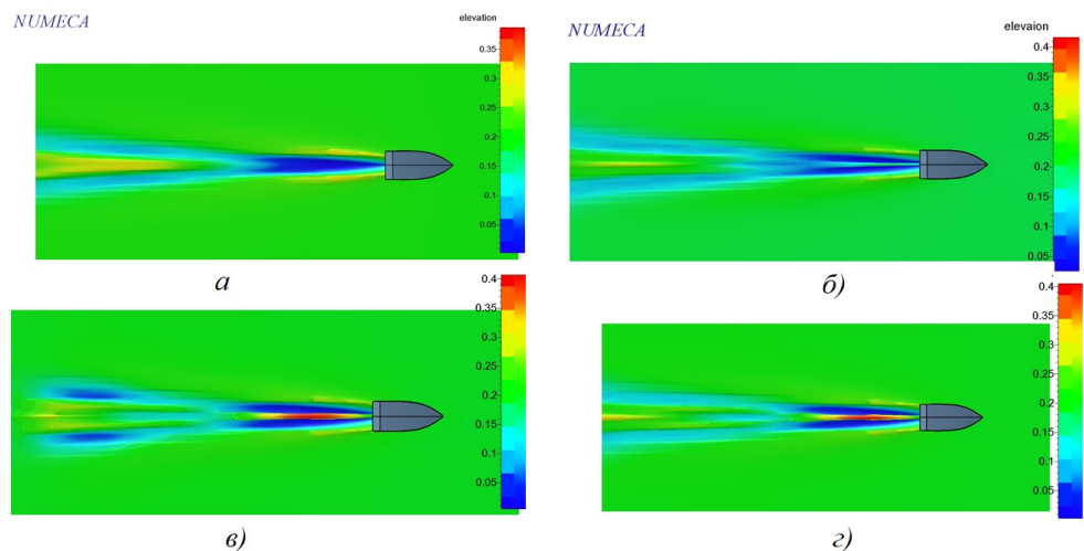
Рис. 14. Волновой след при движении катера со скоростью 22 м/с: а) D=0 мм; б) D=250 мм; в) D=375 мм; г) D=420 мм.
