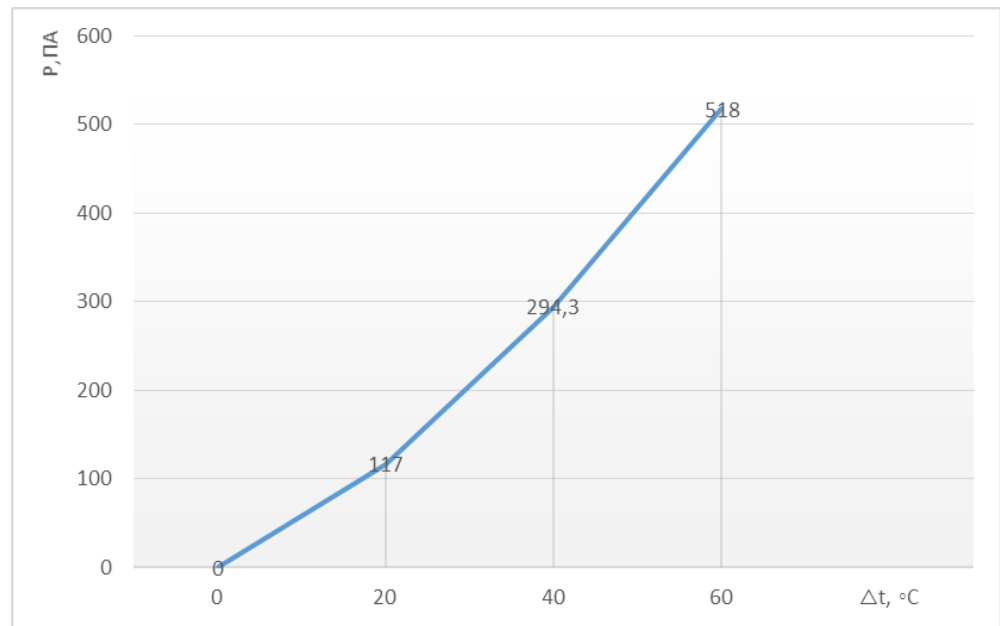
Рис. 4. Напор циркуляции в канале кингстонного ящика
