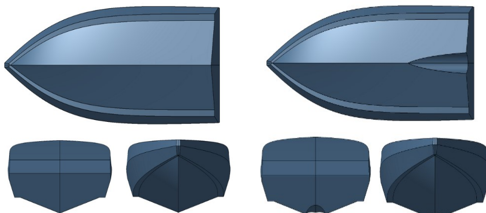
Рис. 2. Геометрия катера. а) исходный корпус; б) корпус с тоннелем D=420 мм.
