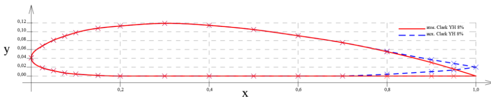
Рис. 1. Исходный (синий) и изменённый (красный) профили Clark YH 8%
