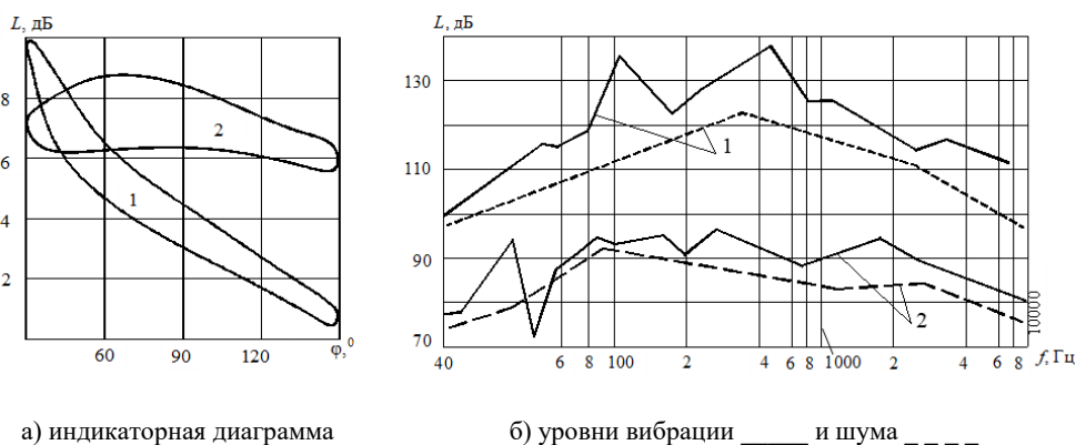
а) индикаторная диаграмма б) уровни вибрации _____ и шума - - - - 1 – дизель; 2 – двигатель Стирлинга Рис. 2. Сравнение характеристик дизеля и двигателя Стирлинга (рисунок автора)
