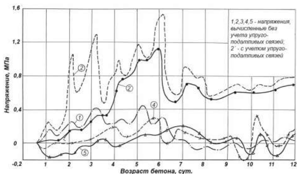
Рис.7. Напряжения в контрфорсе 22 секции Андиганской плотины в строительный период 1,4 – датчики в блоке с поливом; 2, 5 – в блоке без ухода
