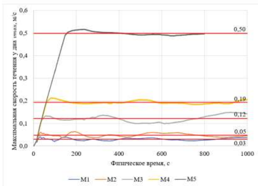
Рис. 4. Графики изменения максимальной скорости течения у дна канала глубиной 10 м
