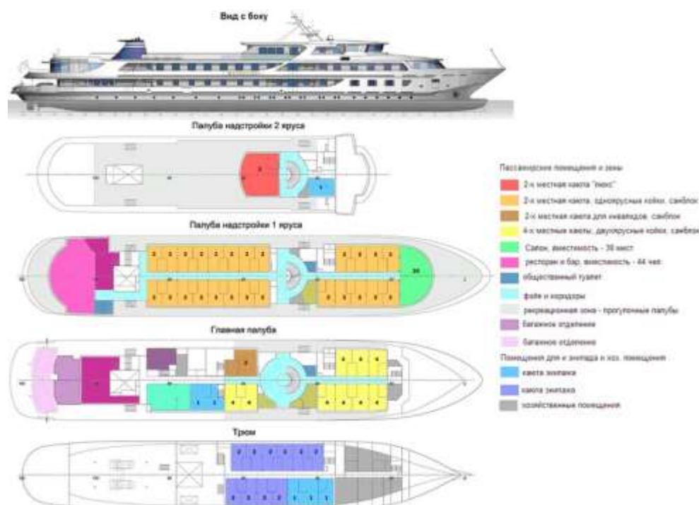
Рис. 1. Круизный теплоход проекта ST12078P
