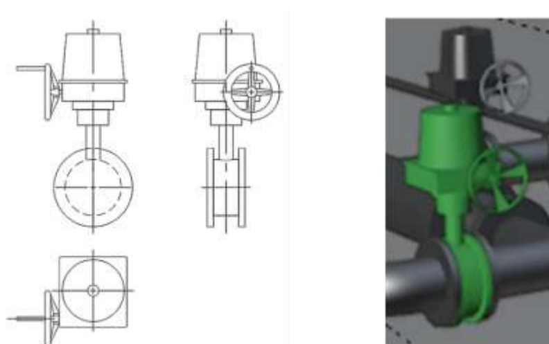
Рис. 5. Эскизы и трехмерная модель поворотного затвора с электроприводом
