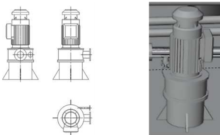
Рис. 3. Эскизы и трехмерная модель двигателя грузового насоса судна
