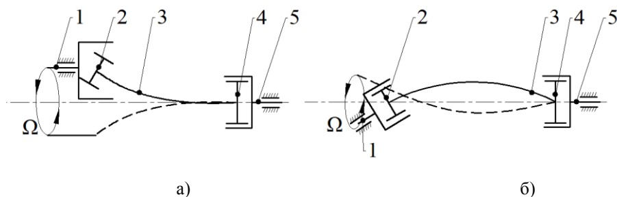
1 – вал; 2, 4 – зубчатые втулки; 3 – рессора; 5 – вал приводного механизма
