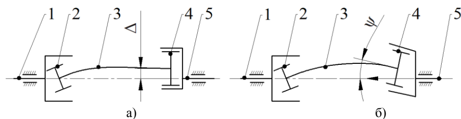
1 – вал двигателя; 2, 4 – зубчатые втулки; 3 – рессора; 5 – вал приводного механизма
