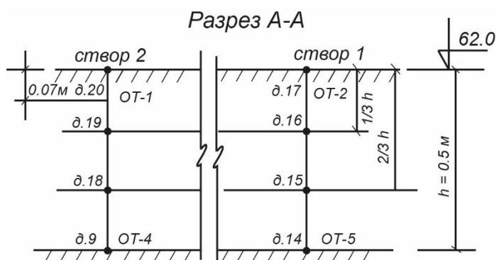
Рис. 6. Схема размещения датчиков температуры и телетензометров, створ 2 – поливы, шатер; створ 1 – без ухода д.20 – датчик температуры №20; Т-2 – телетензометр №2
