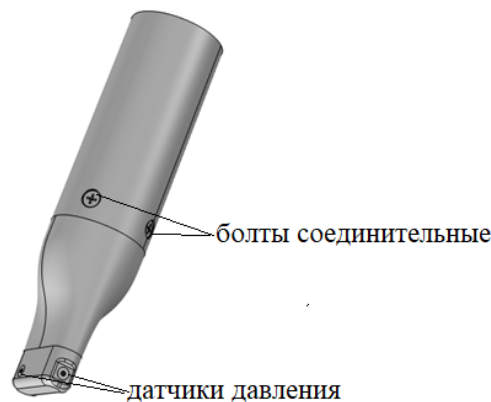
Рис. 3. Модель гидродинамического лага с расположенными датчиками давления
