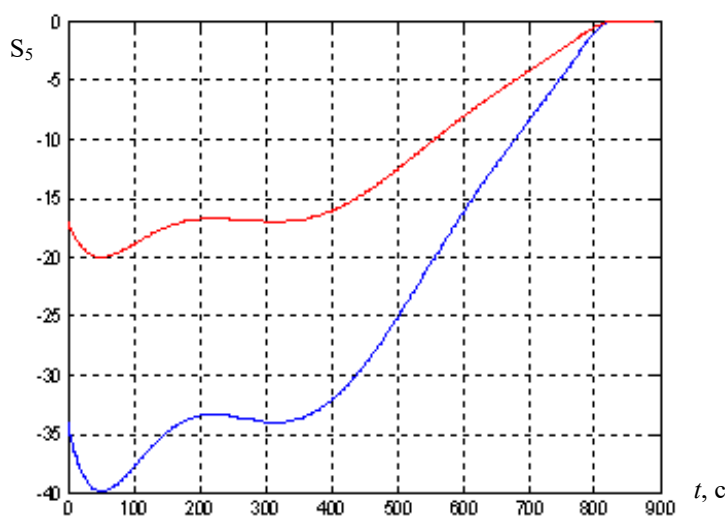
Рис. 3. Коэффициент усиления по курсу
