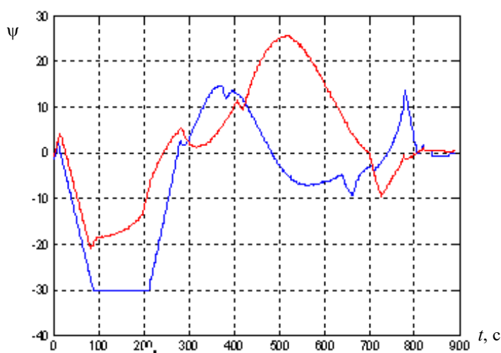
Рис. 4. Угол перекадки руля
