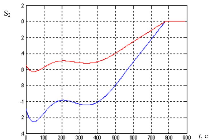
Рис. 1. Коэффициент усиления по положению
