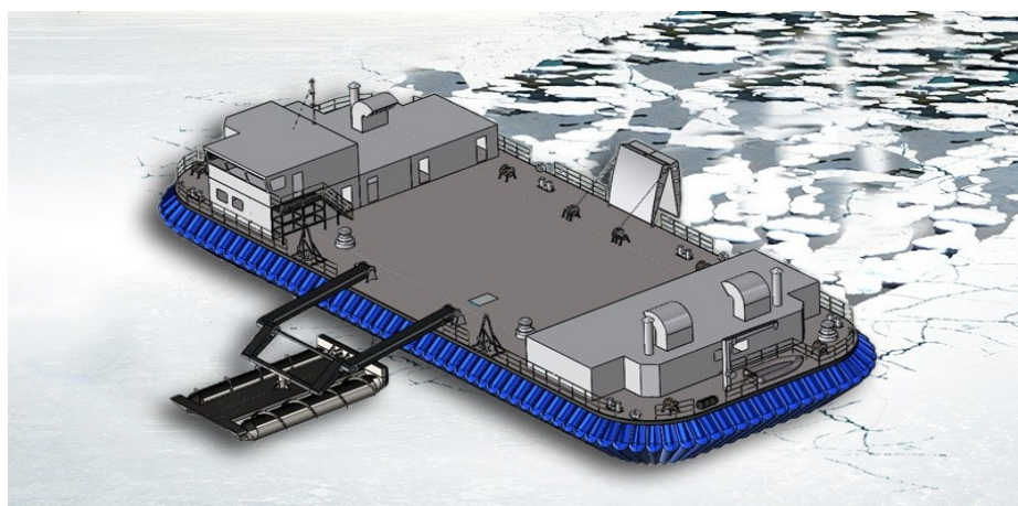
Рис. 1. Архитектурно-конструктивный тип ледокольной платформы на воздушной подушке
