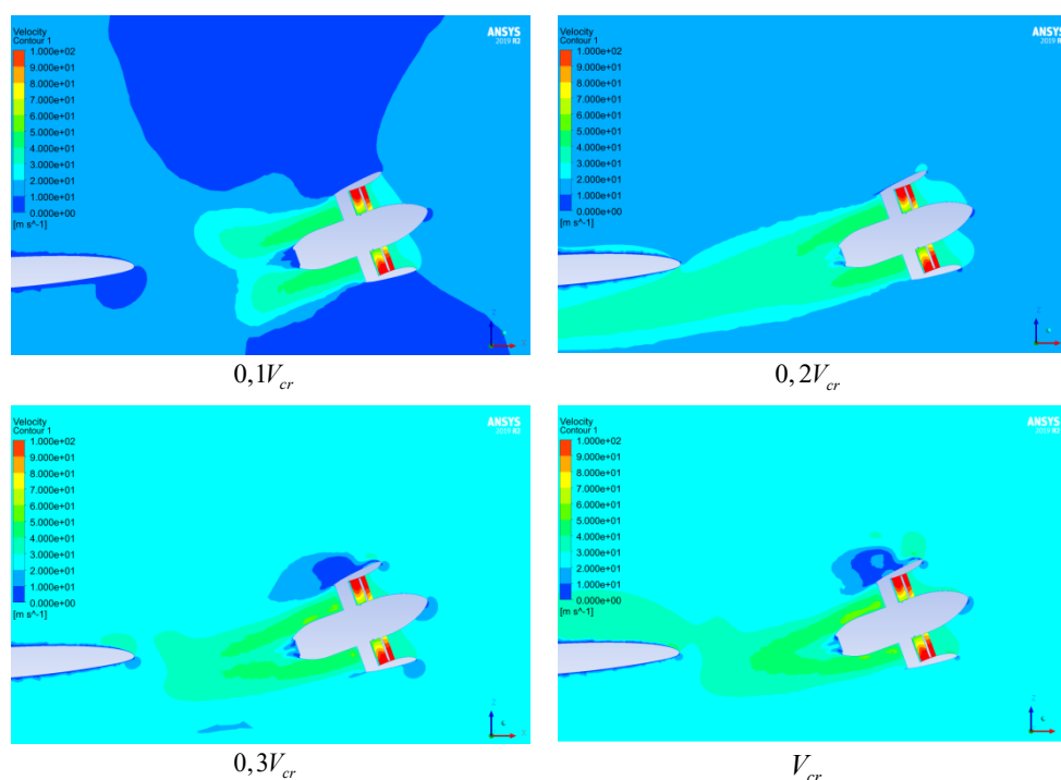
Рис. 6. Диаграммы распределения скорости аэродинамического течения в сечении мидаля поддувного винта, полученные по результатам численного моделирования для разных скоростей движения
