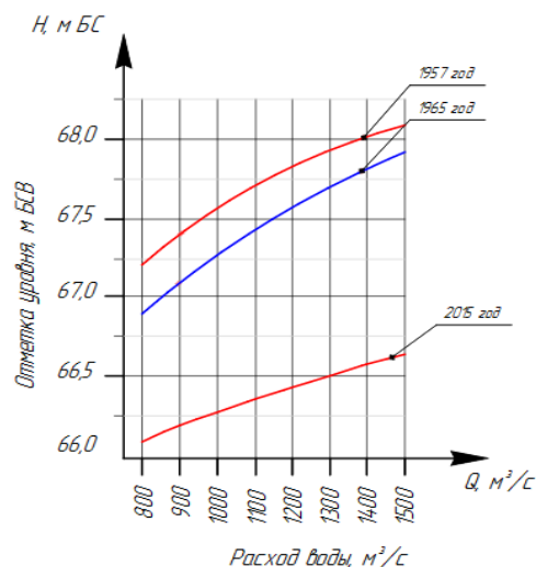
Рис. 3. Динамика изменения графика связи расхода от уровня воды по гидropосту №7 в течение ряда лет
