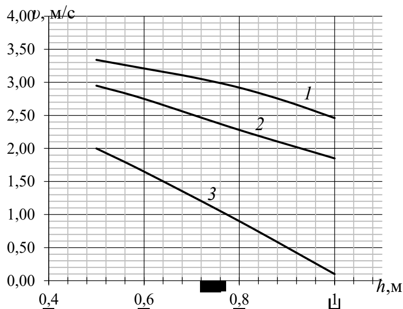
Рис. 6. Диаграммы ледопроеходимости: 1 – ЛПВП с РВД; 2 – состав ЛПВП и буксир проекта ПЕ65; 3 – состав ЛПВП и ледокол «Капитан Измайлов»
