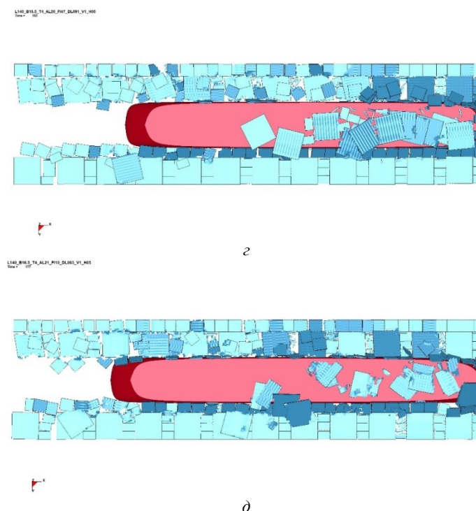
Рис. 2. Характер «обтекания» ледяной средой судовых корпусов различных габаритов и форм: а – V-образная форма судна; длина 80 м; ширина 10 м; осадка 1,5 м; коэффициент носовой полноты водоизмещения 0,62; угол наклона форштевня 16 градусов; угол наклона ватерлинии 30 градусов; б – традиционная форма судна; длина 80 м; ширина 10 м; осадка 1,5 м; коэффициент носовой полноты водоизмещения 0,91; угол наклона форштевня 16 градусов; угол наклона ватерлинии 38 градусов; в – судно с тупым носовым бульбом; длина 80 м; ширина 10 м; осадка 1,5 м; коэффициент носовой полноты водоизмещения 0,94; угол наклона форштевня – 64 градуса; угол наклона ватерлинии 29 градусов; г – традиционная форма судна; длина 140 м; ширина 16,5 м; осадка 4 м; коэффициент носовой полноты водоизмещения 0,91; угол наклона форштевня 47 градусов; угол наклона ватерлинии 20 градусов; д – традиционная форма судна; длина 140 м; ширина 16,5 м; осадка 4 м; коэффициент носовой полноты водоизмещения 0,93; угол наклона форштевня 10 градусов; угол наклона ватерлинии 21 градус
