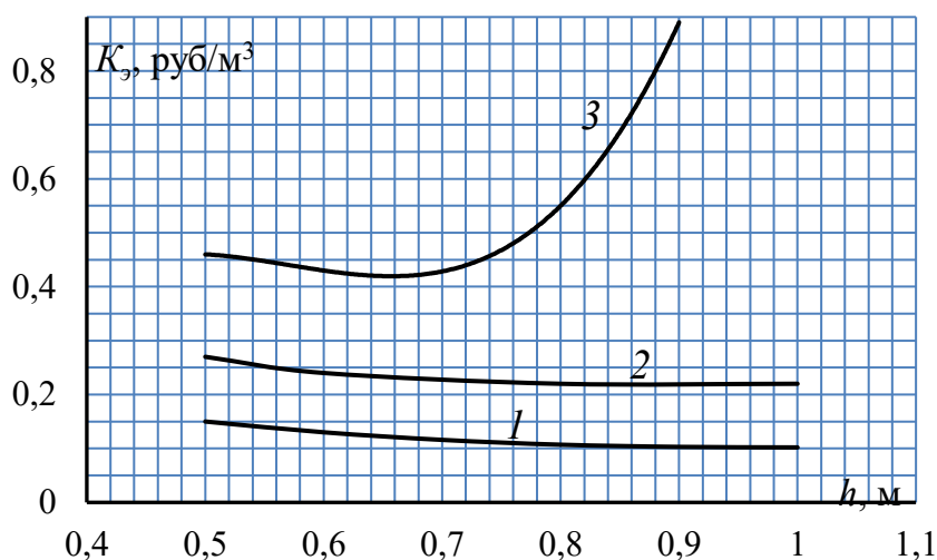
Рис. 8. Экономическая эффективность прокладки ледового канала: 1 – ЛПВП с РВД; 2 – состав ЛПВП и буксир проекта ПЕ65; 3 – состав ЛПВП и ледокол «Капитан Измайлов»
